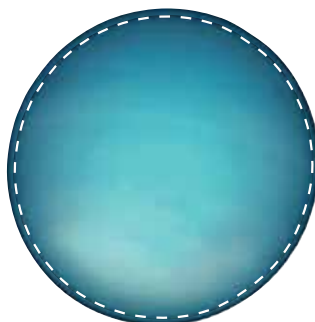
Uranus
