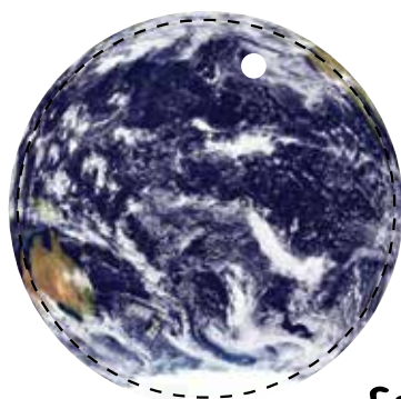
Earth
